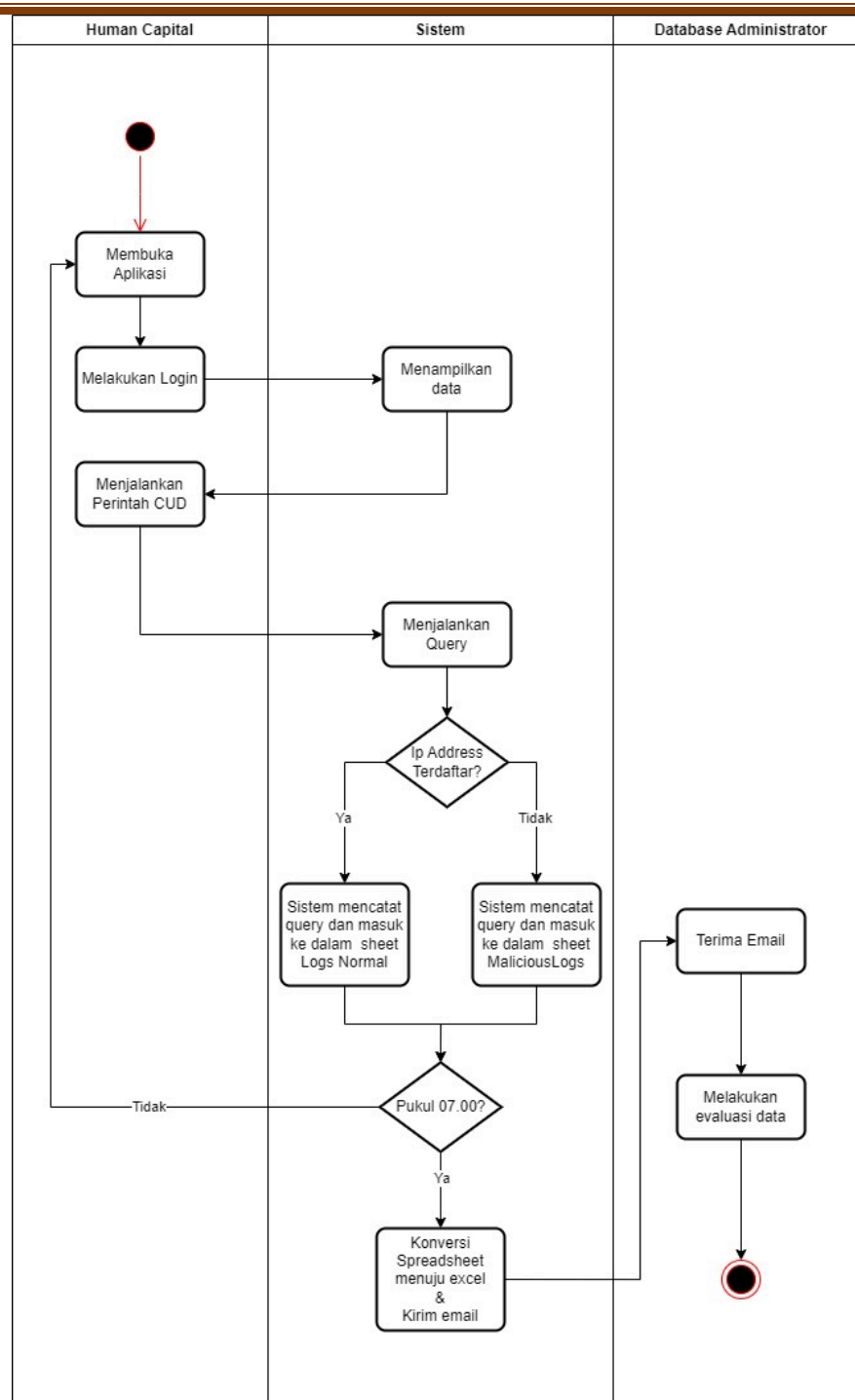
Gambar 2. Diagram Aktivitas
